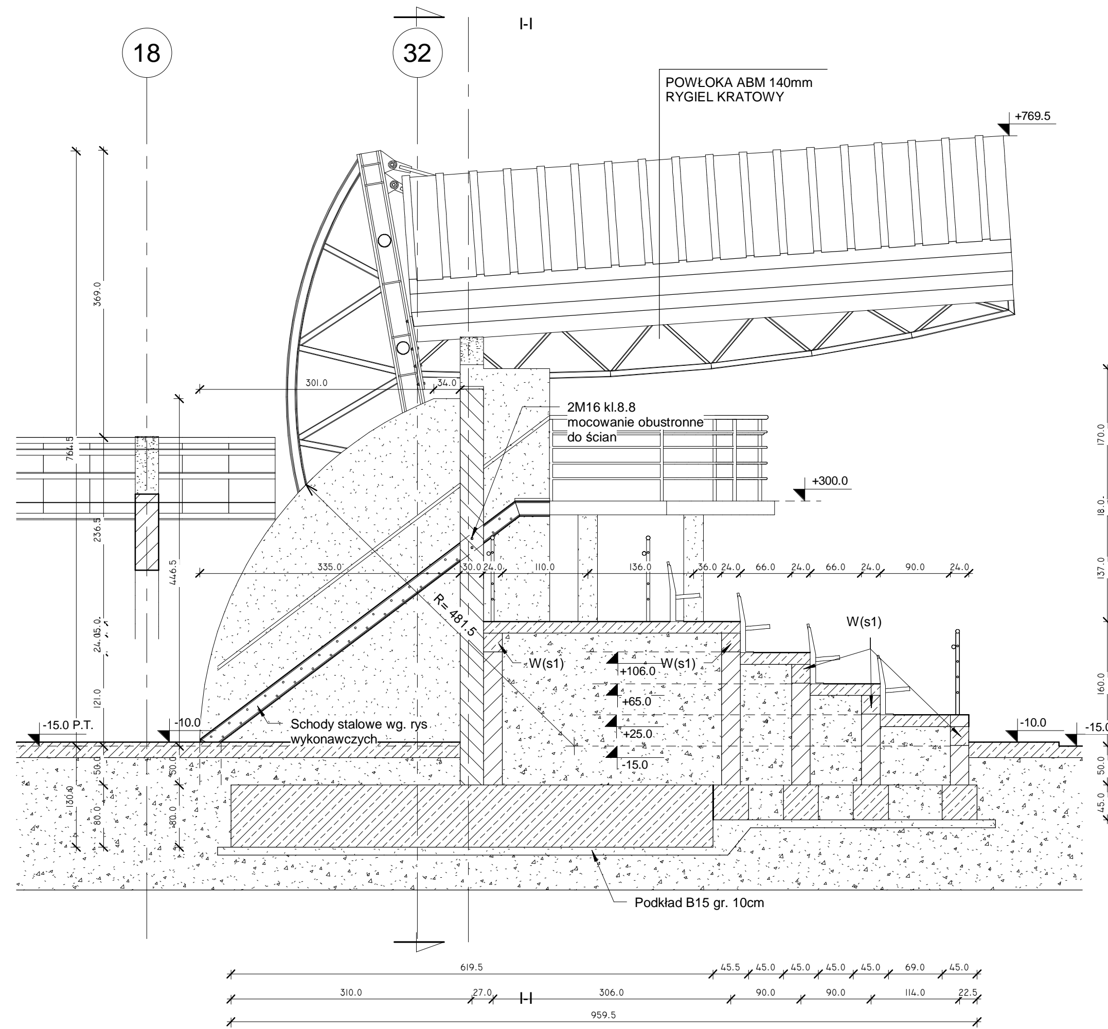
1 J-J 1:50
