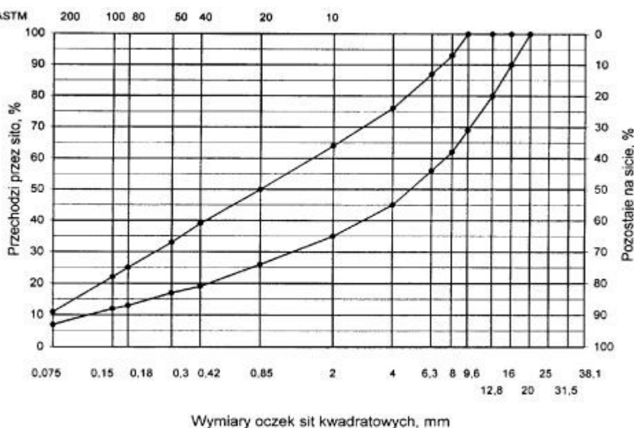
Rys. 1. Krzywe graniczne uziarnienia mieszanki mineralnej BA od 0 do 16mm do warstwy ścieralnej nawierzchni drogi o obciążeniu ruchem KR 1-2
