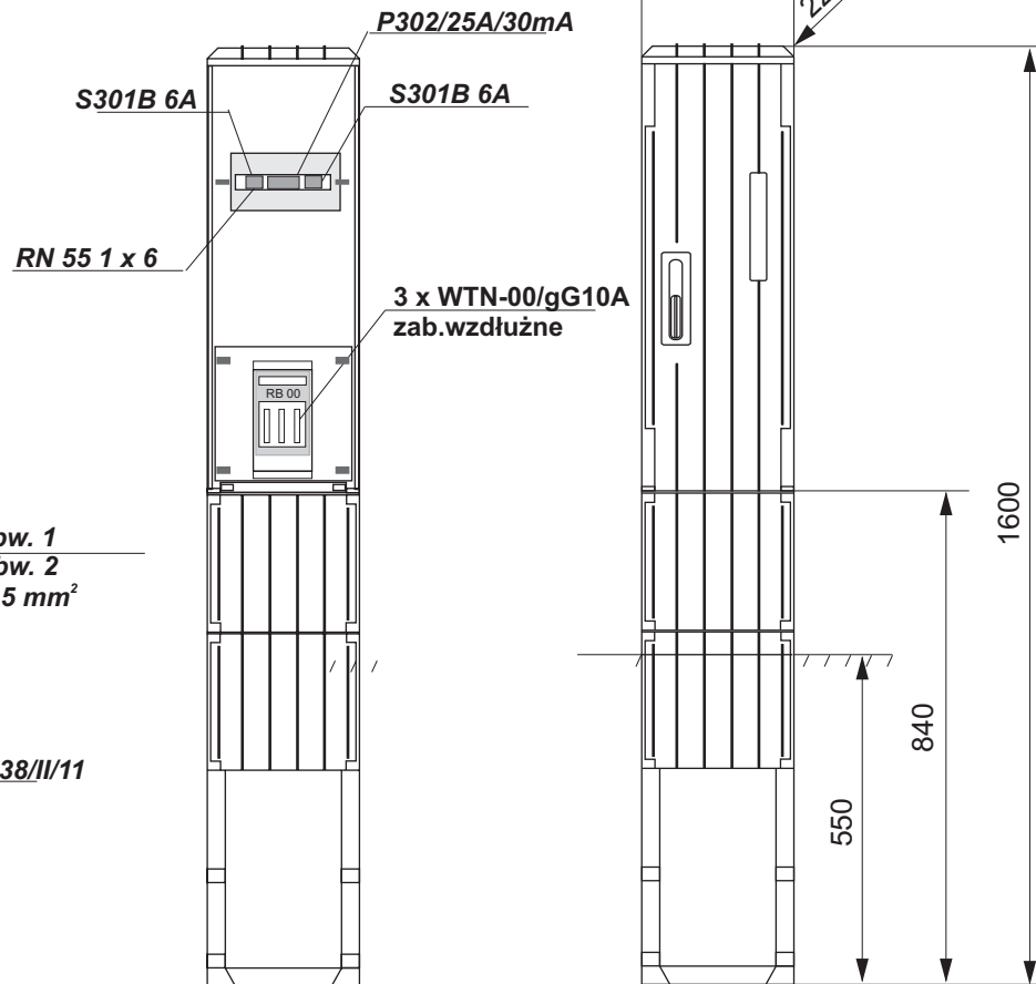
Szafa zasilania oświetlenia zabudowanego na moście
