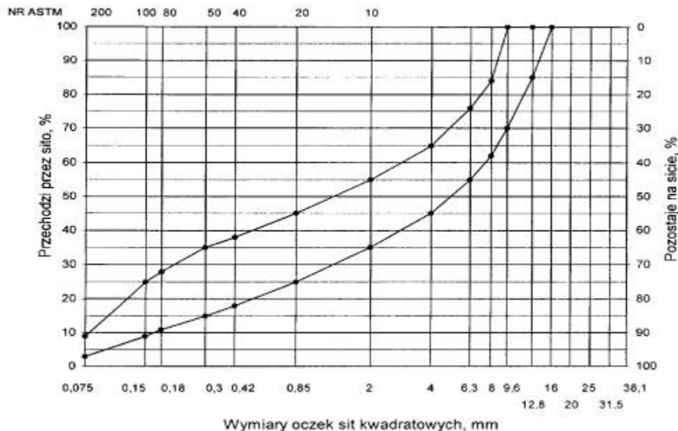
Rys. 1. Krzywe graniczne uziarnienia mieszanki mineralnej BA od 0 do 12,8 mm do warstwy wiążącej nawierzchni drogi o obciążeniu ruchem KR 1-2
