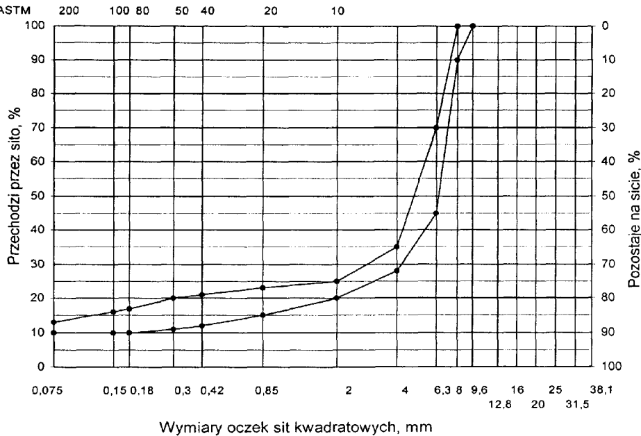
Rys. 4. Krzywe graniczne uziarnienia mieszanki mineralnych SMA od 0 mm do 8,00 mm KR1-2
