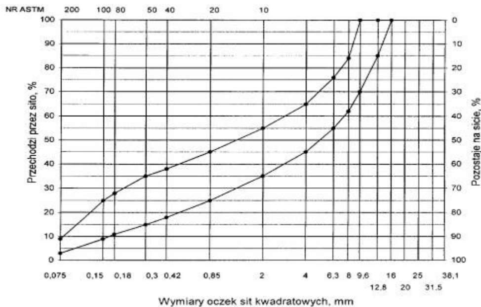
Rys. 1. Krzywe graniczne uziarnienia mieszanki mineralnej BA od 0 do 20 mm do warstwy wyrównawczej nawierzchni drogi o obciążeniu ruchem KR 1-2
