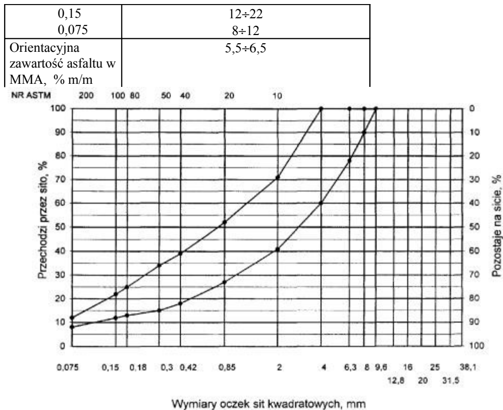
Rys. 1. Krzywe graniczne uziarnienia mieszanki mineralnej BA od 0 do 6,3 mm do warstwy wyrównawczej nawierzchni drogi o obciążeniu ruchem KR 1-2
